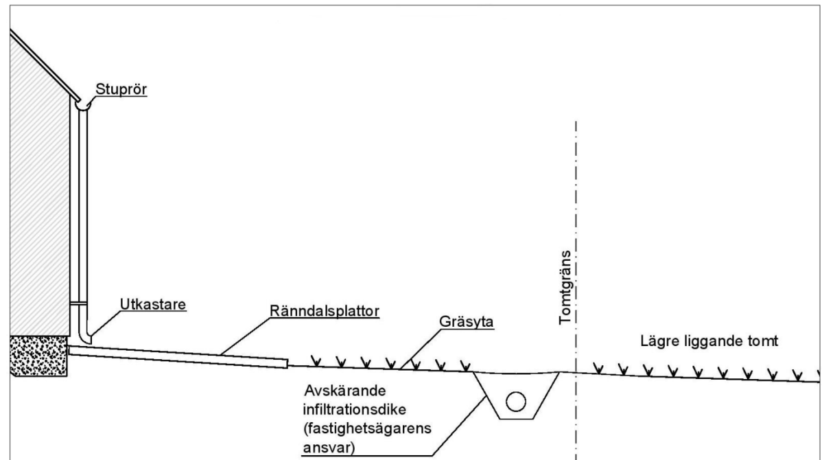
Figur 14 Till höger. Principskiss över avskärande dike vid fastighetsgräns för att skydda intilliggande tomt från ytligt rinnande dagvatten. (AH Vattenlogik, 2016)
